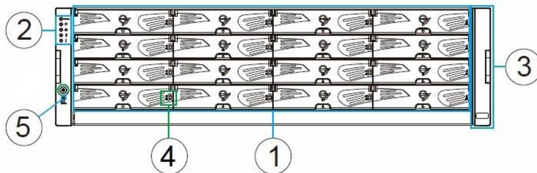
图 1- 3.GS5316D 前视图组件分布
