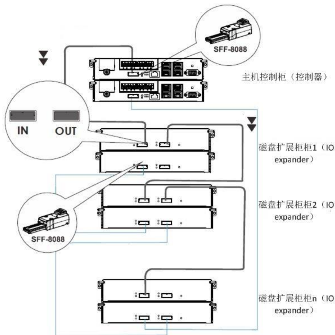
图 1-7.GS5316D 扩展柜连接示意图
